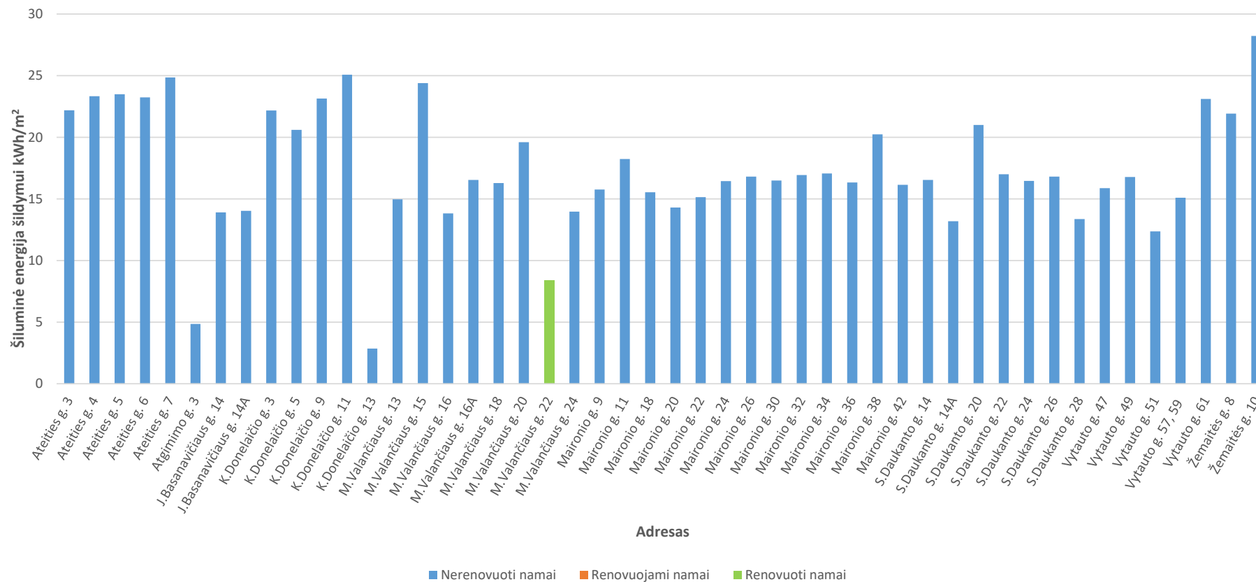
2019m. gruodžio mėn. gyvenamųjų namų šiluminės energijos suvartojimas šildymui kWh/m 2
